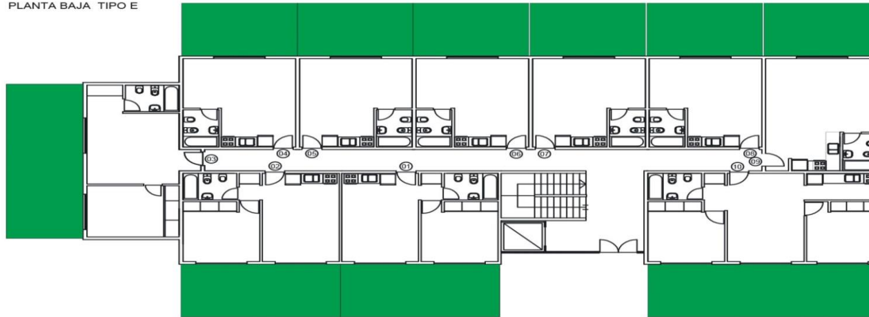
PLANTA BAJA TIPO E
