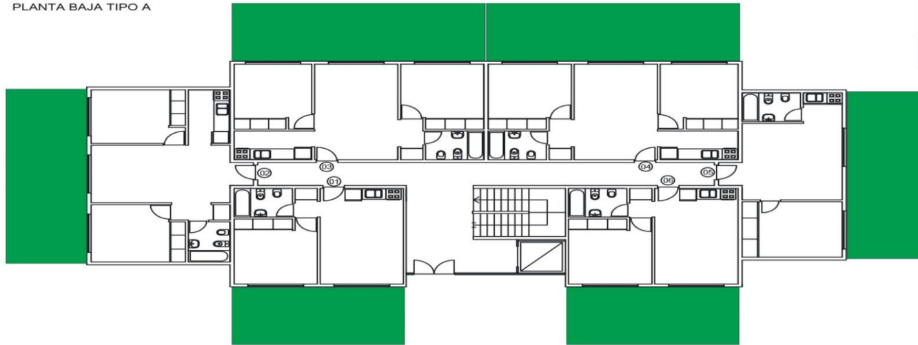
PLANTA BAJA TIPO A
