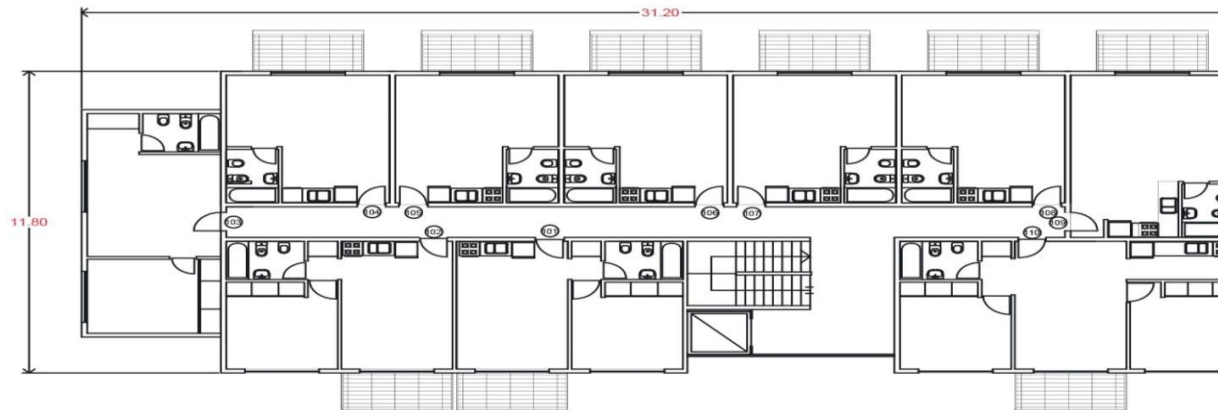
PLANTA ALTA TIPO E
