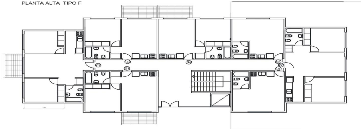
PLANTA ALTA TIPO F
