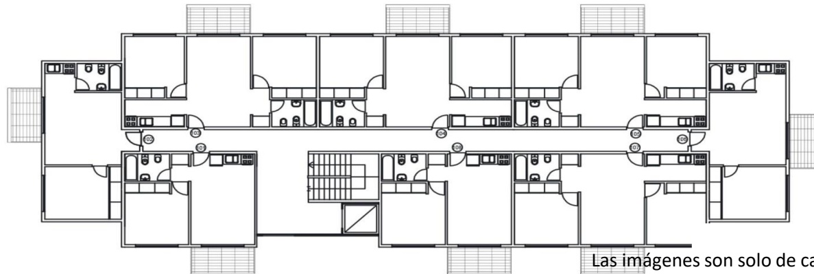
PLANTA ALTA TIPO B
